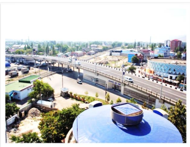
Махачкалинский путепровод
